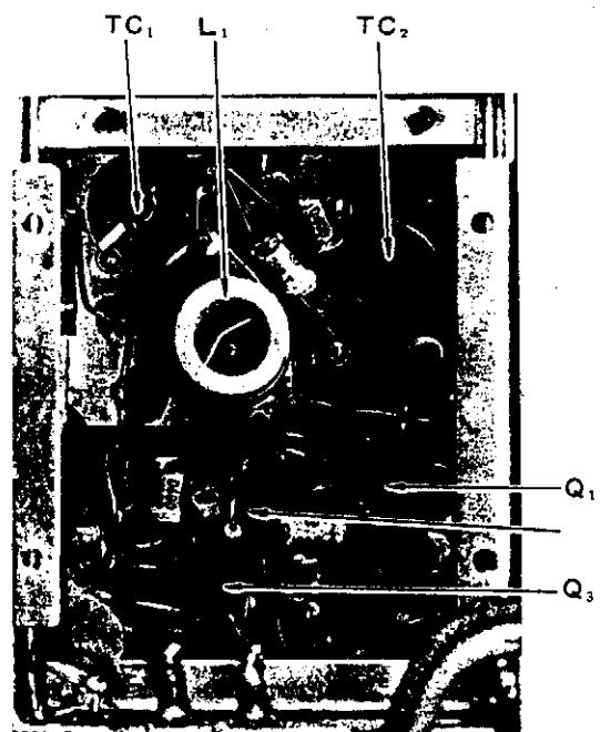
VFO Module
